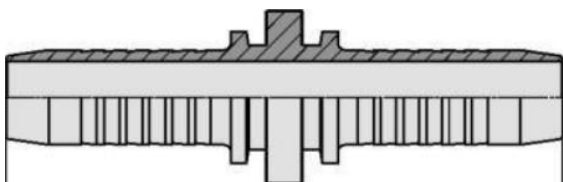
CONECTOR ESPIGA DOBLE (cod.DES) 1/4 - 3/8 - 1/2 - 5/8 - 3/4 - 1 pulgada
