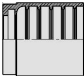
CAMISA PARA MANGUERA HIDRÁULICA DOBLE MALLA (cod.CDM) 1/4 - 3/8 - 1/2 - 5/8 - 3/4 - 1 pulgada
