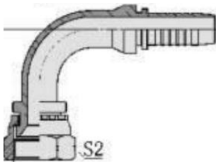
HEMBRA GIRATORIA CODO NF (cod.HGN) Ver hoja de precios para tamaños
